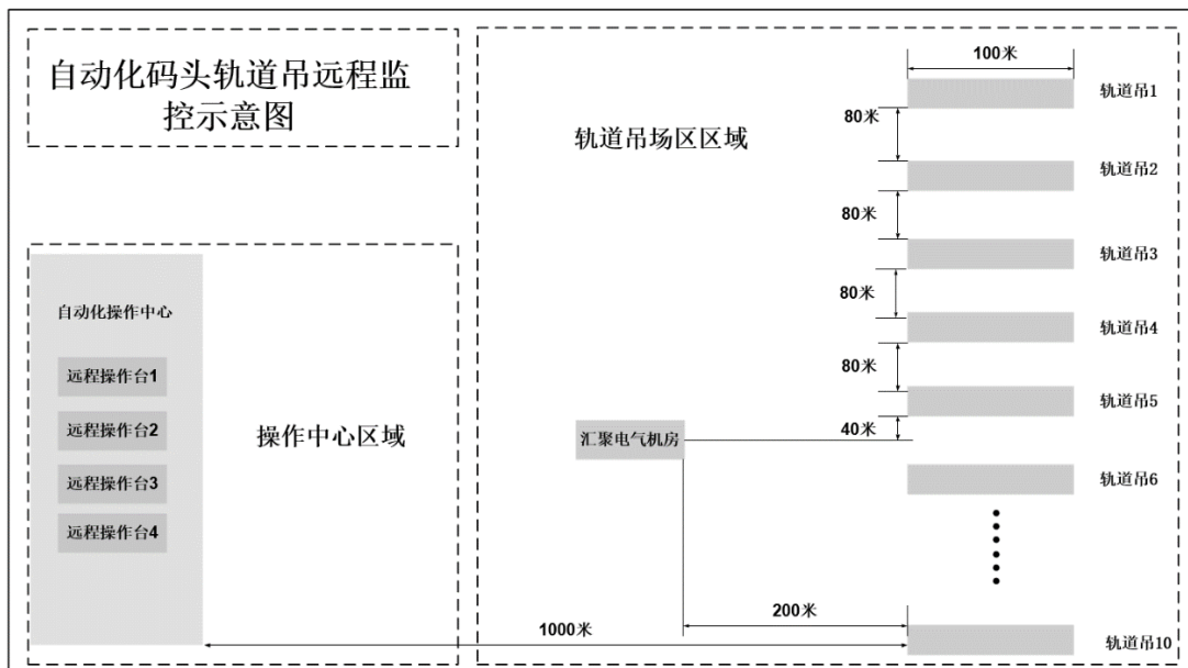
图 2 项目布置示意图
