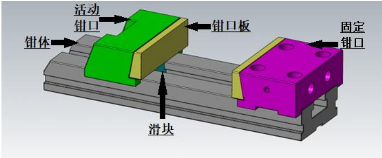
附件 3.1 精密平口钳总装配图：
