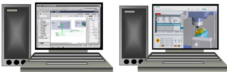
图 3 数控数字化双胞胎虚拟调试赛项配套任务平台 TIA Portal 和 Create My Virtual Machine
