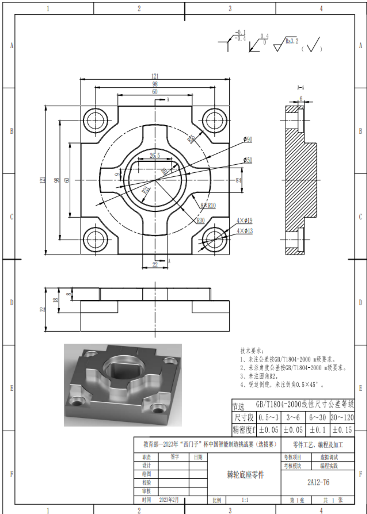
附件 2 样件零件图
