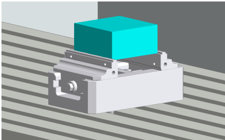
图 7 正确安装工装体
