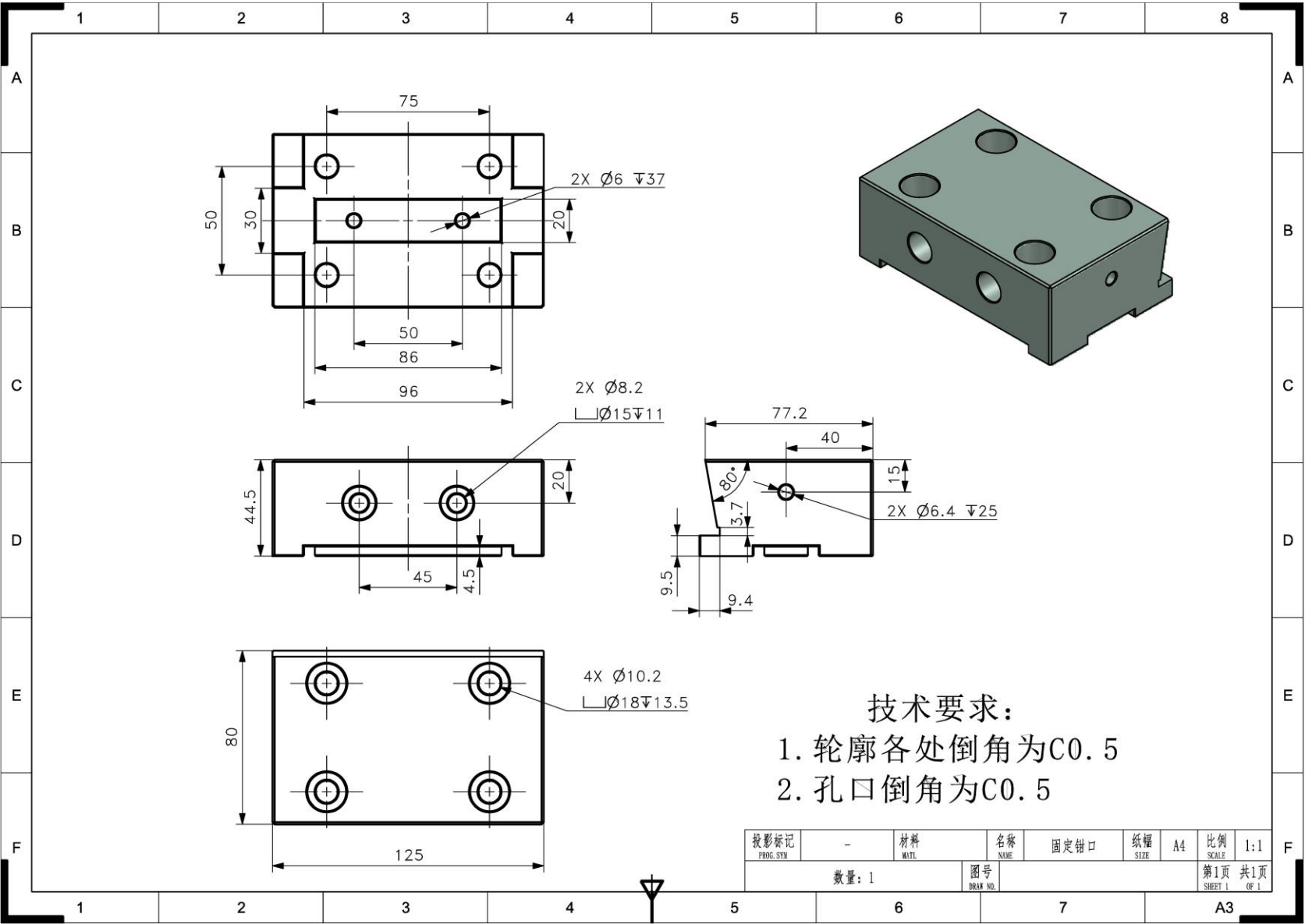
附件 3.3 固定钳口零件图：
