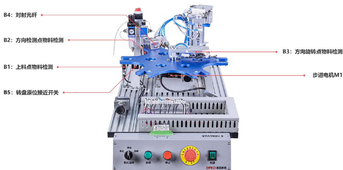
图 8 旋转工作站主视图 2
